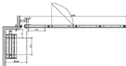
Dvoubodové zavěšení
